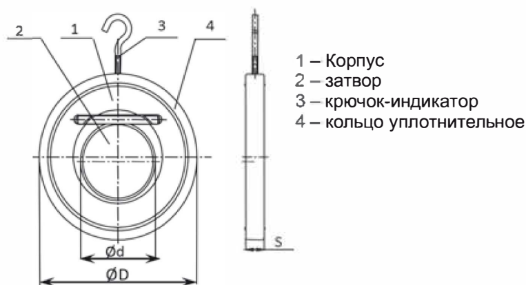
Рисунок 1 Общий вид клапанов обратных
