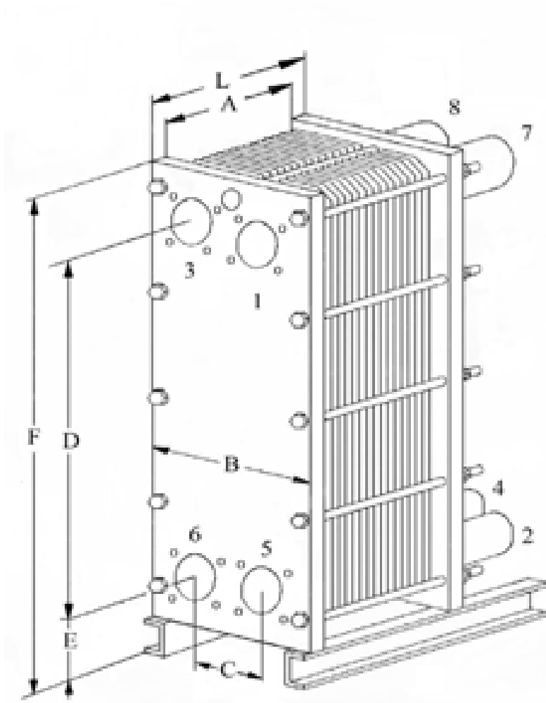
Рис.4. Схема трехходового теплообменника ТР:
